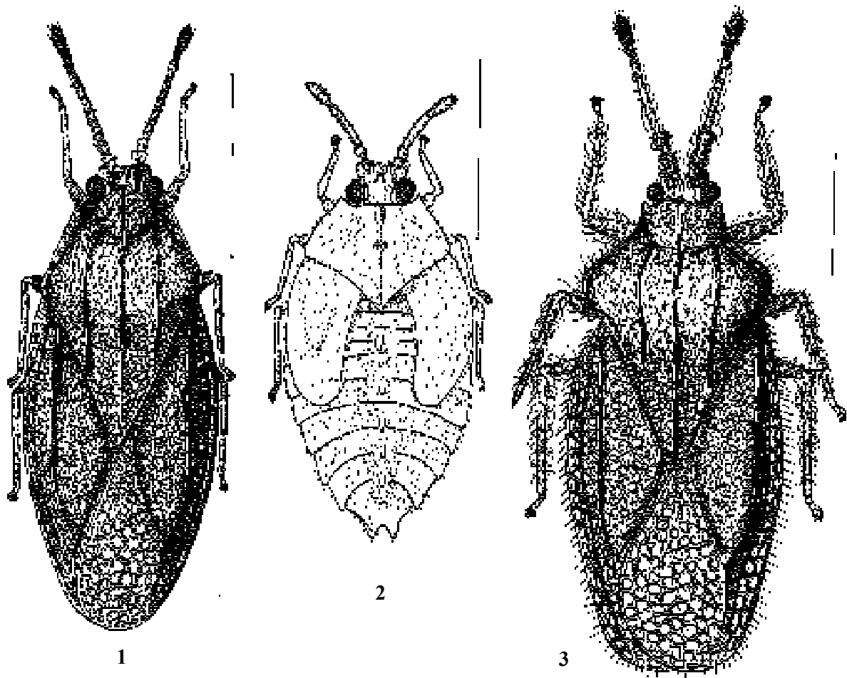
Рис. 1–3. Габитус, сверху: 1–2 — Tingis (Tingis) kerzbnieri sp.n.; 3 — T. (Tropidocheila) afemeljanovi sp.n.; 1, 3 — имаго; 2 — личинка 5-го возраста. Масштаб — 1 мм.
